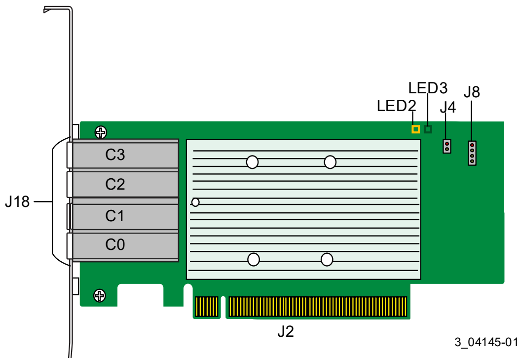
Abbildung 1 Aufbau der Karte für den ThinkSystem 440-16e SAS/SATA 12-Gbit-Adapter
