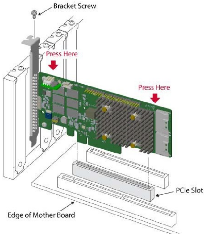
Abbildung 2 Installation eines Adapters in einem PCIe-Steckplatz
