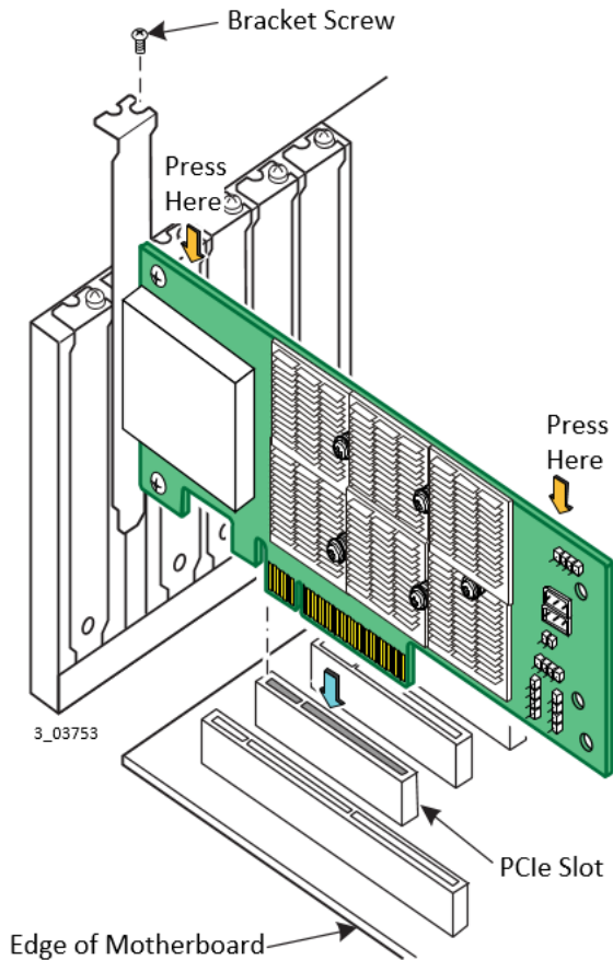
Figura 2 Instalación de un adaptador en una ranura de PCIe
