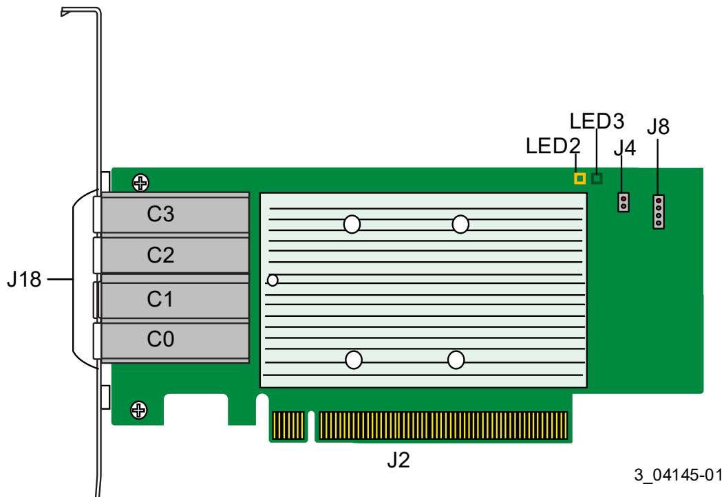
Figura 1 Diseño de tarjeta para el adaptador ThinkSystem 440-16e SAS/SATA 12Gb
