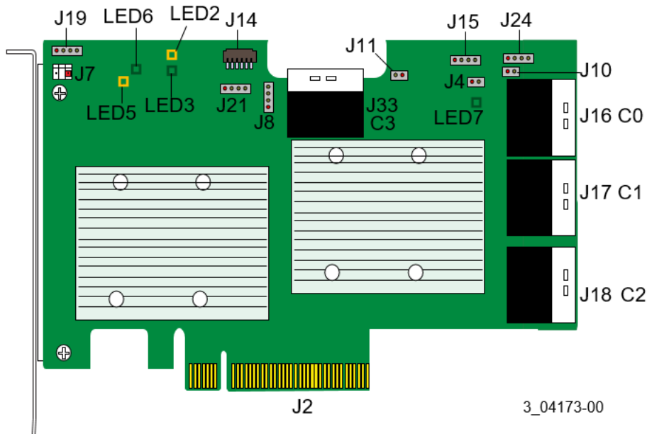
Figura 1 Diseño de tarjeta para el adaptador ThinkSystem RAID 940-32i 8 GB Flash PCIe Gen4
