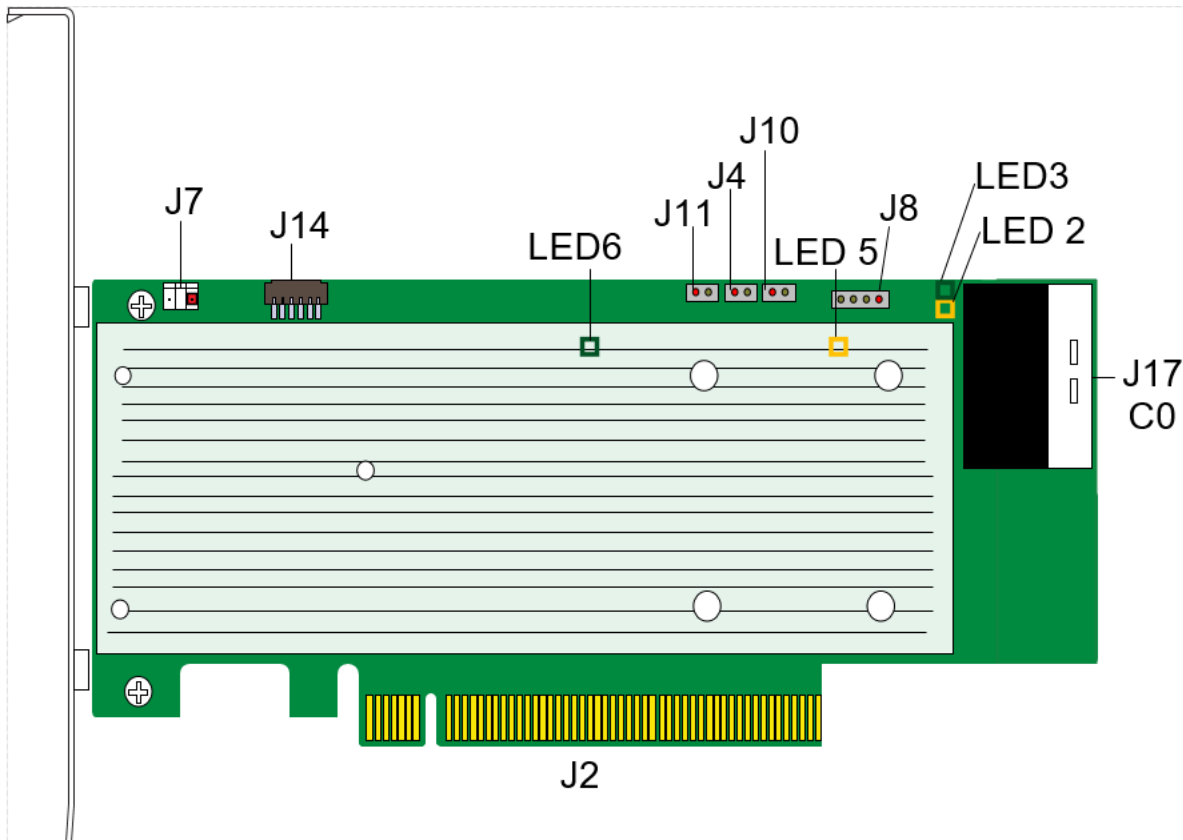
Figura 1 Diseño de tarjeta para el adaptador ThinkSystem RAID 940-8i 8 GB Flash PCIe 12 GB
