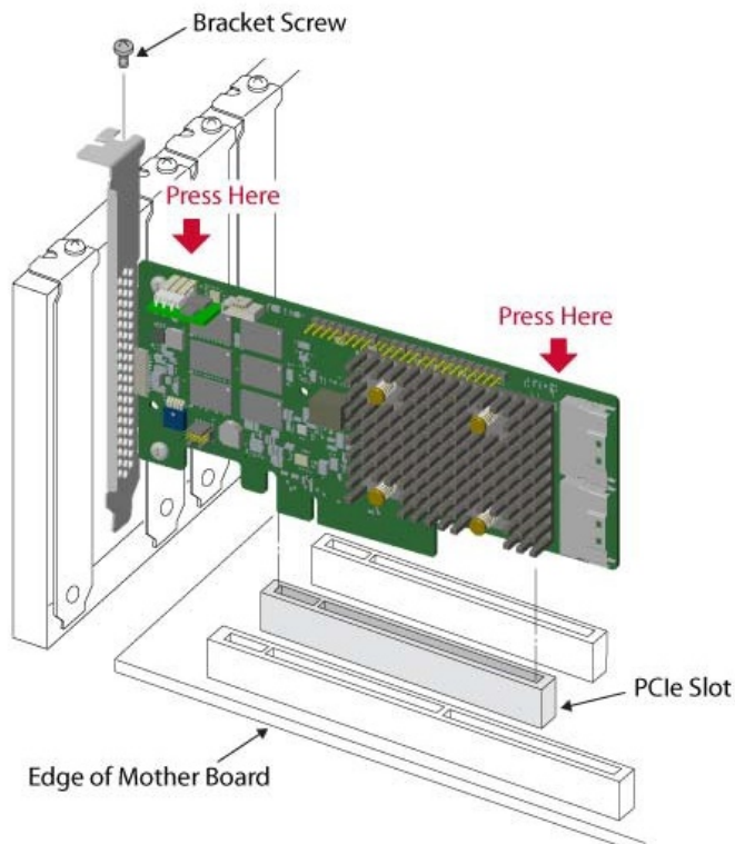
Figure 2 Installation d'un adaptateur dans un emplacement PCIe
