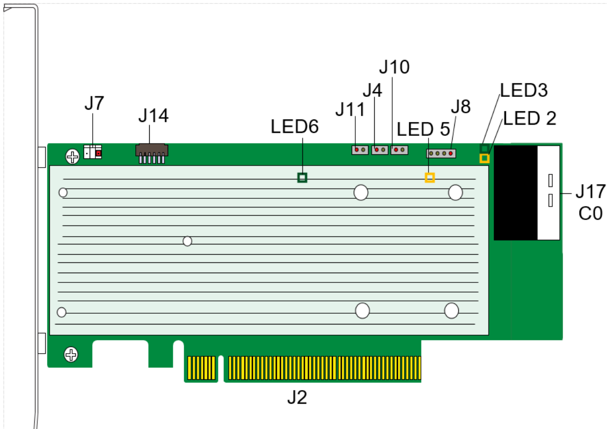
Figure 1 Disposition de la carte pour l'adaptateur ThinkSystem RAID 940-8i mémoire Flash 8 Go PCIe 12 Gb
