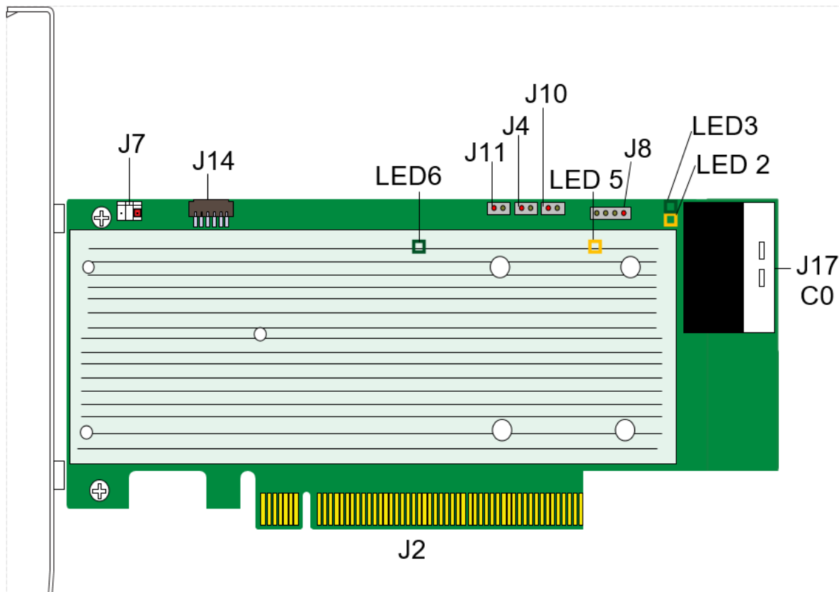
Figura 1 Layout della scheda per l'adattatore Thinksystem RAID 940-8i 8GB Flash PCIe da 12 Gb
