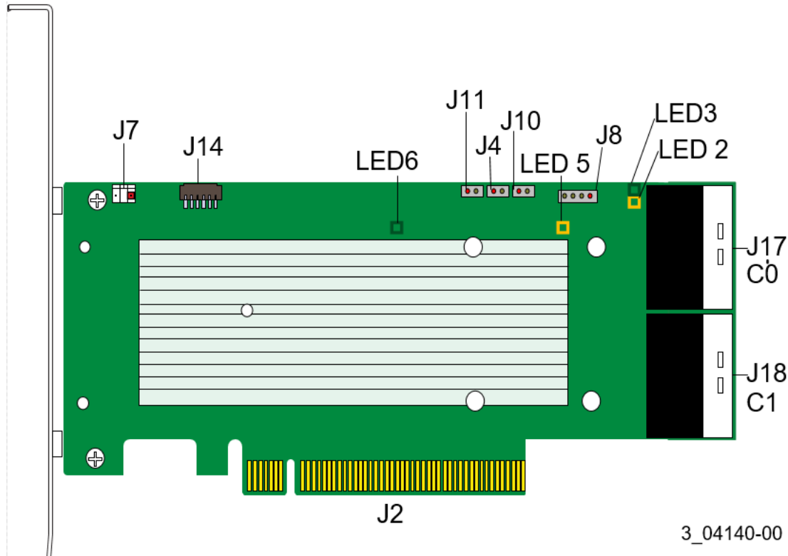
図 1 ThinkSystem RAID 940-16i 8GB フラッシュ PCIe Gen4 アダプターのカードのレイアウト
