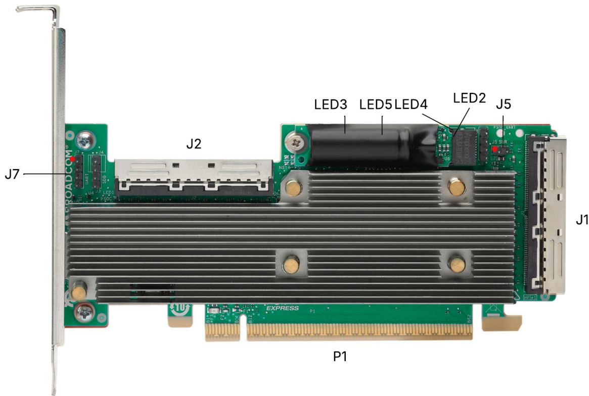
図 1: ThinkSystem RAID 960W-32i PCIe Gen5 24Gb Adapter のカードのレイアウト
