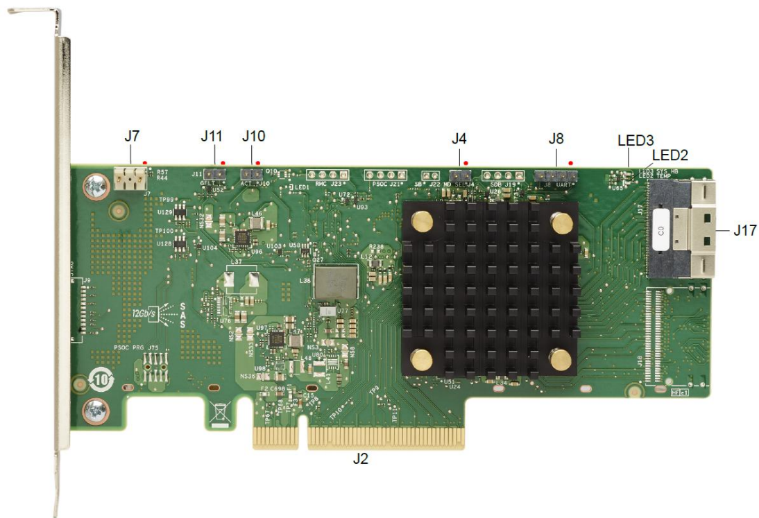
図 1: ThinkSystem RAID 545-8i PCIe Gen4 12Gb Adapter のカードのレイアウト
