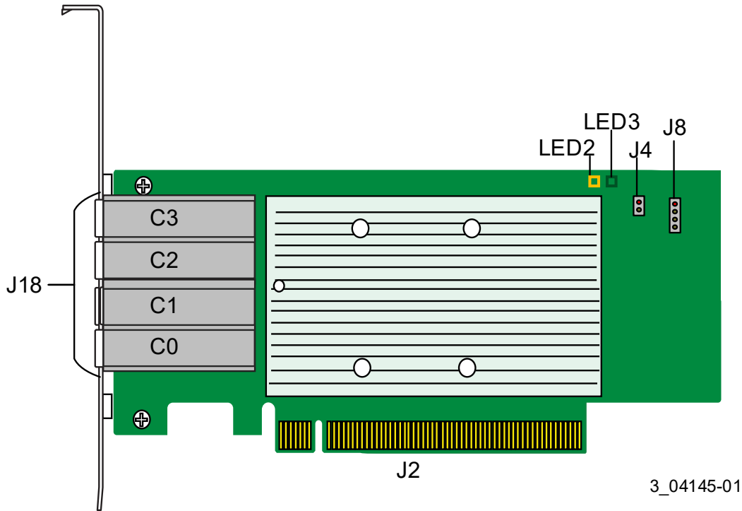
그림 1 ThinkSystem 440-16e SAS/SATA 12Gb 어댑터의 카드 레이아웃
