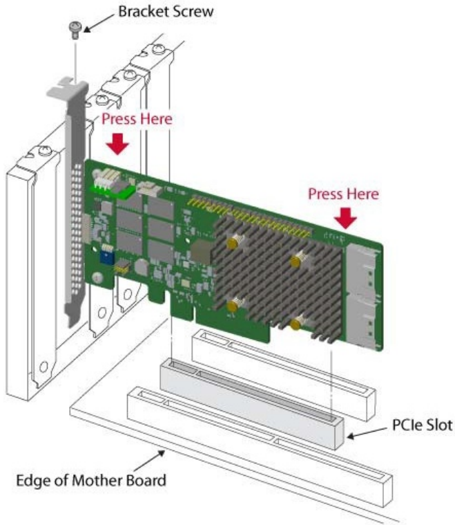
그림 2 PCIe 슬롯에 어댑터 설치
