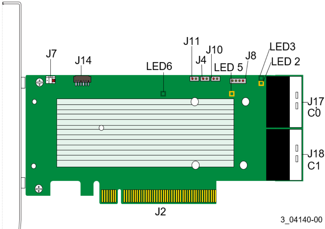
그림 1 ThinkSystem RAID 940-16i 8GB 플래시 PCIe Gen4 어댑터의 카드 레이아웃
