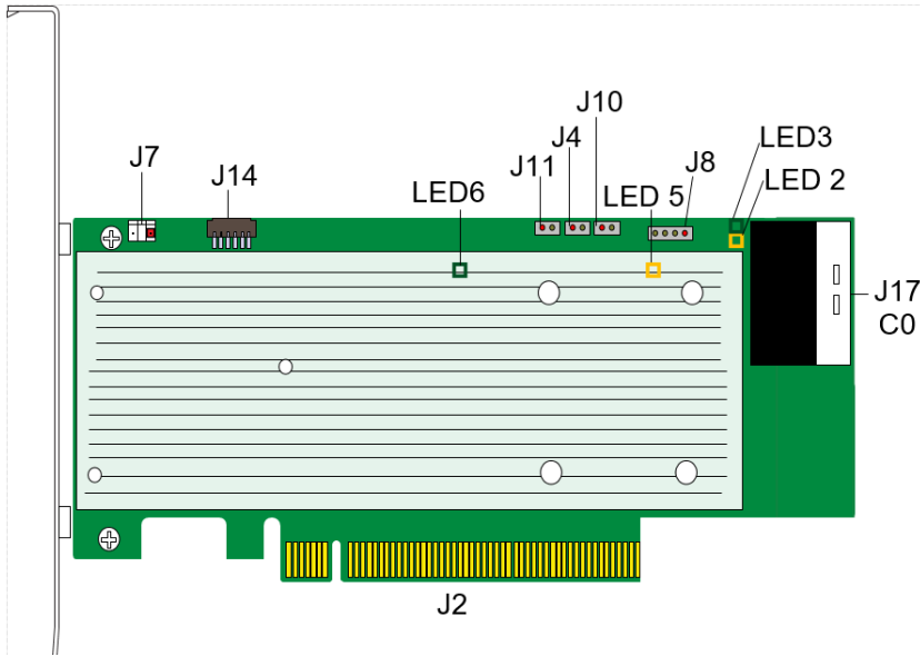
그림 1 ThinkSystem RAID 940-8i 4GB 플래시 PCIe Gen4 12Gb 어댑터의 카드 레이아웃
