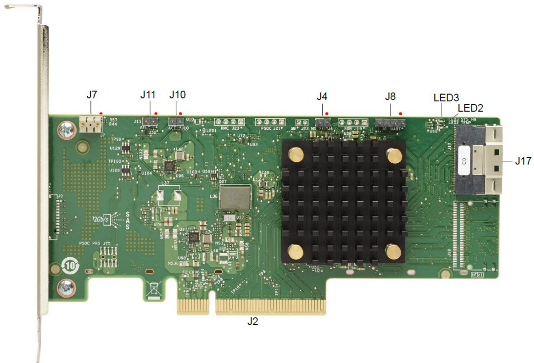
그림 1: ThinkSystem RAID 545-8i PCIe Gen4 12Gb Adapter의 카드 레이아웃
