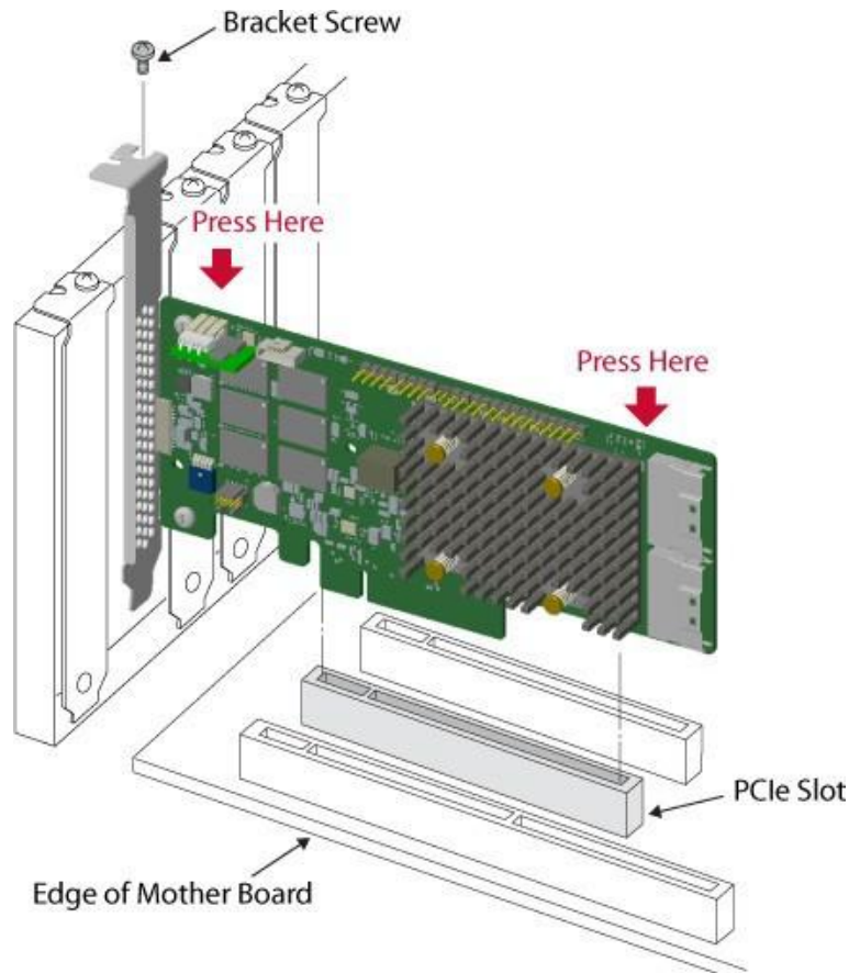
그림 2: PCIe 슬롯에 어댑터 설치
