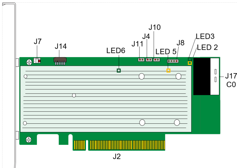
Figura 1 Layout da placa do adaptador ThinkSystem RAID 940-8i de 4 GB Flash PCIe Gen4 de 12 Gb
