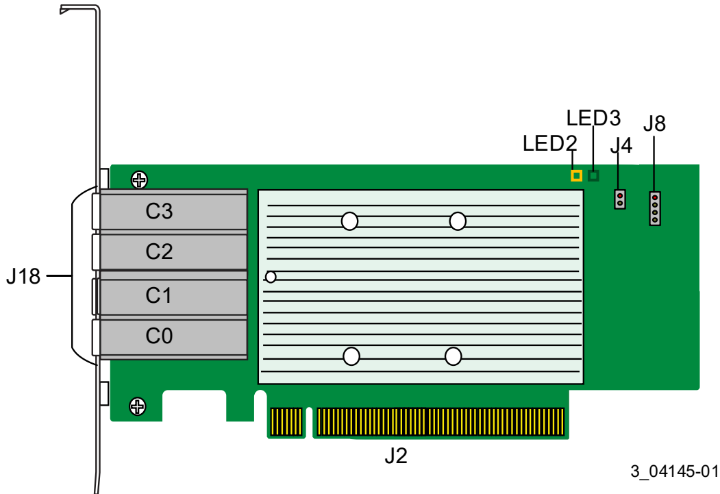
Рис. 1 Компоновка платы для адаптера Thinksystem 440-16e SAS/SATA 12 Гб
