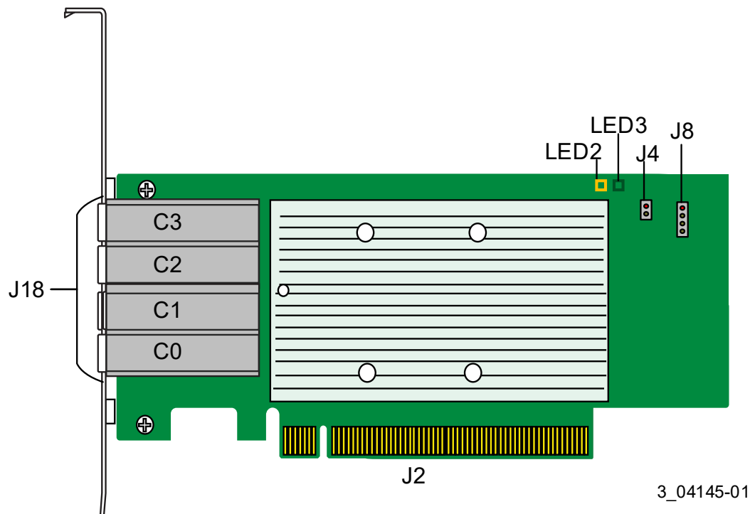
圖例 1 ThinkSystem 440-16e SAS/SATA 12Gb 配接卡的卡片佈置
