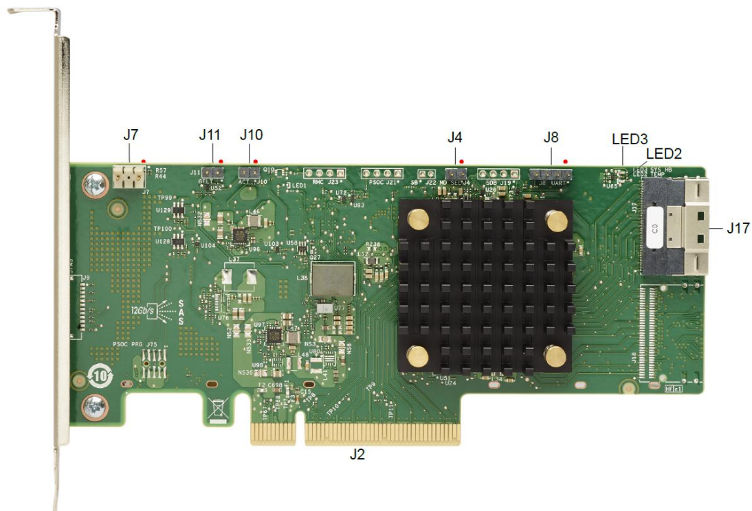
圖 1：ThinkSystem RAID 545-8i PCIe Gen4 12Gb Adapter 的卡片配置
